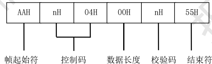
图D.17 请求帧（5）格式
