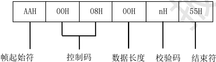
图D.25 请求帧（9）格式
