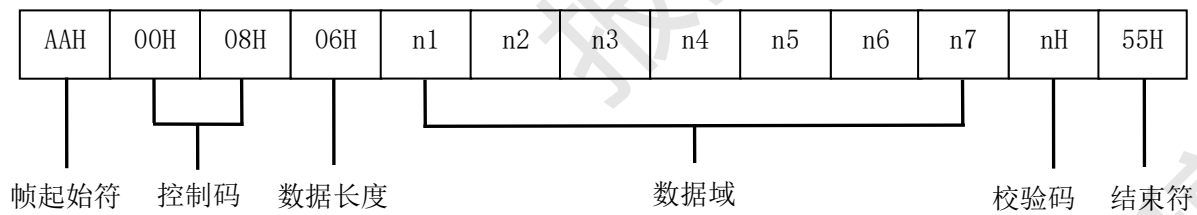
图D. 26 应答帧（9）格式
