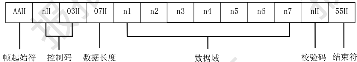
图D.16 应答帧（4）格式
