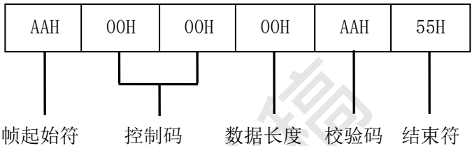
图D.4 请求帧（1）格式
