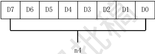
图D.9 月字节格式
