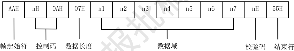
图D. 30 应答帧（11）格式
