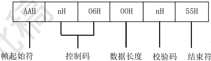
图D.21 请求帧（7）格式
