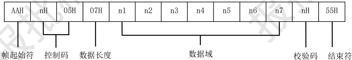
图D.20 应答帧（6）格式
