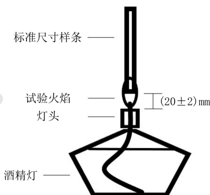
图 C.1 外壳燃烧性能试验示意图 (标准尺寸样条)
