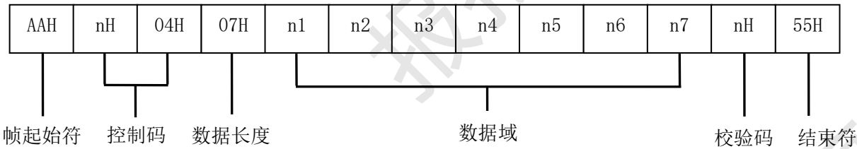
图D.18 应答帧（5）格式
