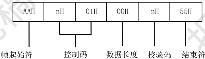
图D. 6 请求帧（2）格式
