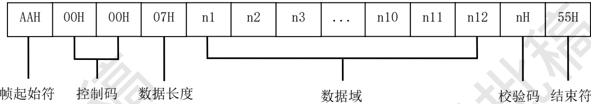
图D.5 应答帧（1）格式
