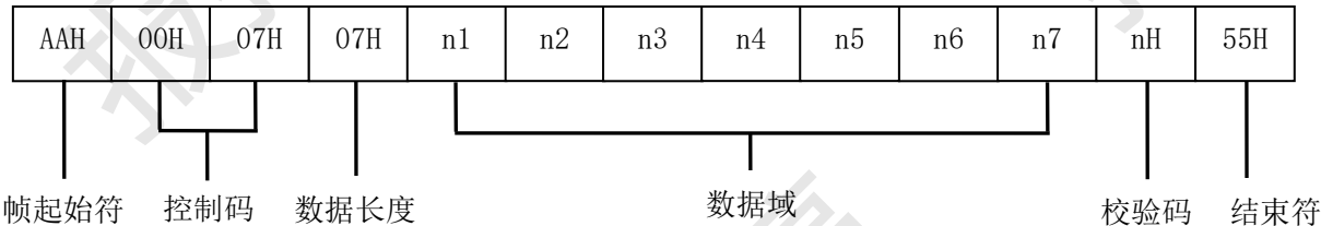
图D.24 应答帧（8）格式
