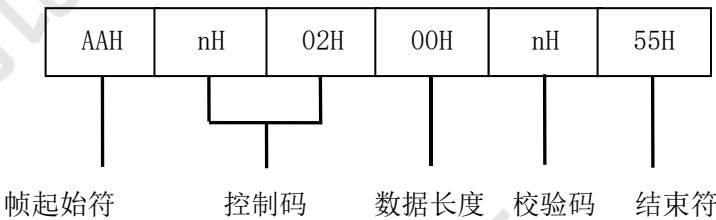
图D.13 请求帧（3）格式
