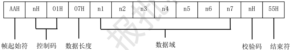
图D. 7 应答帧（2）格式
