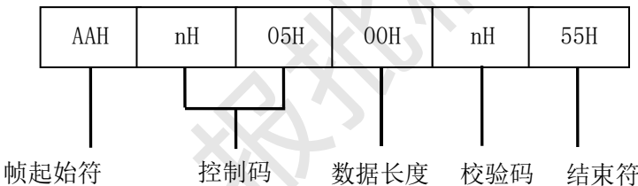
图D.19 请求帧（6）格式
