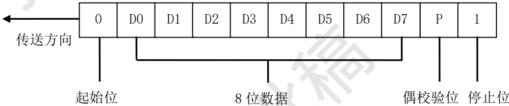
图 D.1 字节传输序列
