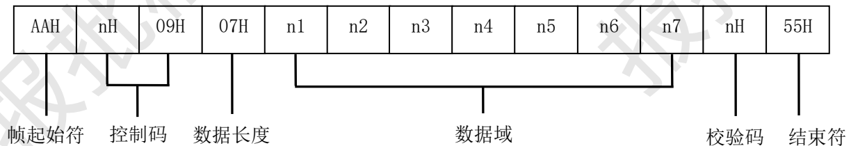
图D. 28 应答帧（10）格式
