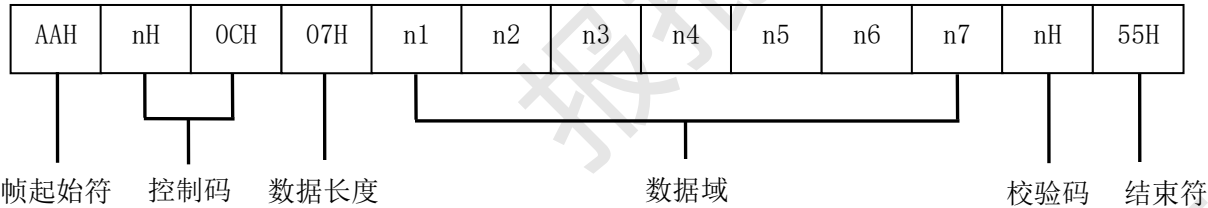
图D. 34 应答帧（13）格式
