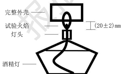
图 C.2 外壳燃烧性能试验示意图 (完整外壳)
