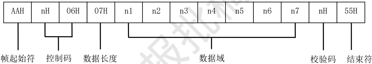
图D.22 应答帧（7）格式
