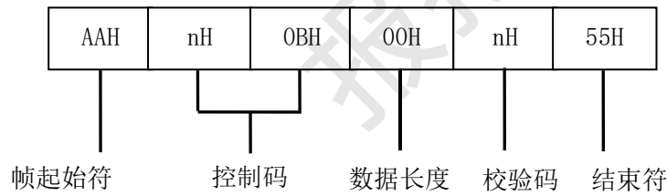
图D.31 请求帧（12）格式
