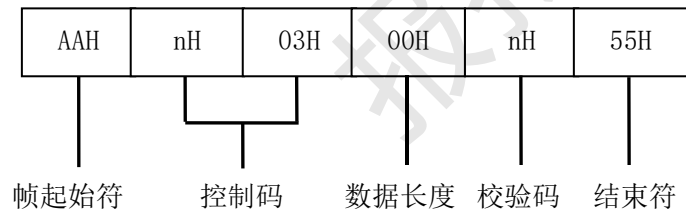
图D.15 请求帧（4）格式
