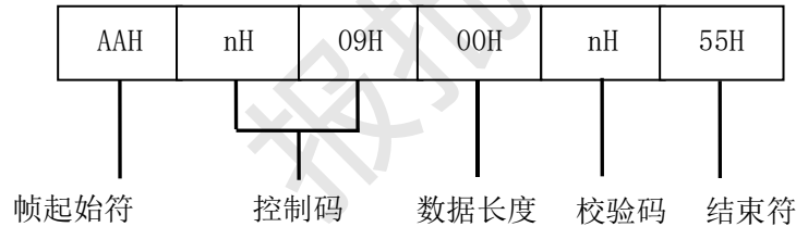
图D. 27 请求帧（10）格式
