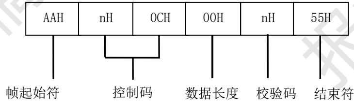
图D.33 请求帧（13）格式
