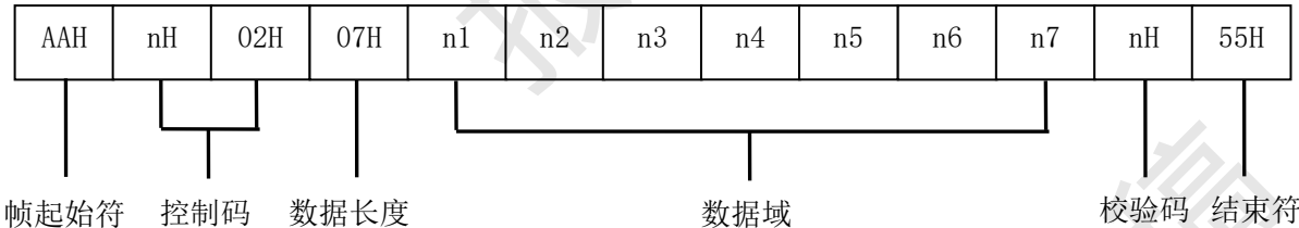
图D.14 应答帧（3）格式
