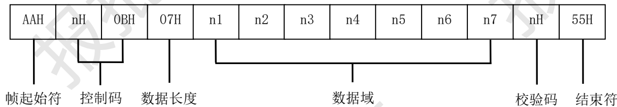
图D.32 应答帧（12）格式
