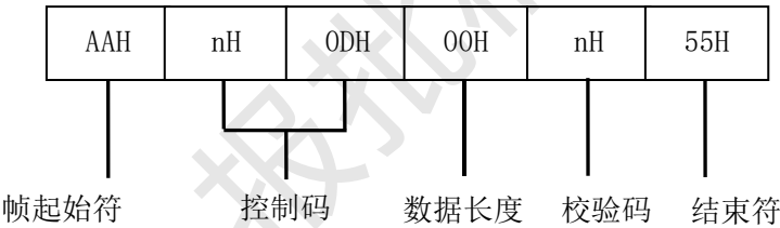
图D. 35 请求帧（14）格式
