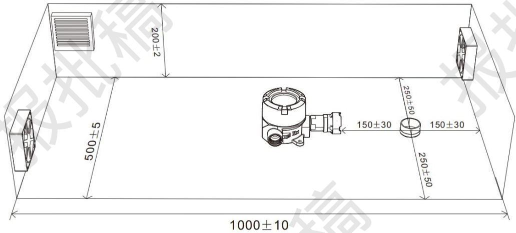
图 B.3 使用液态试剂时的试验布置示意图
