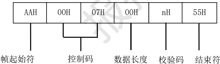
图D.23 请求帧（8）格式
