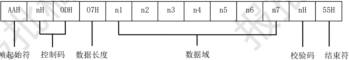
图D. 36 应答帧（14）格式
