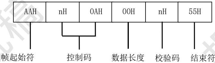
图D. 29 请求帧（11）格式
